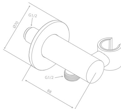
Käsisuihkun pidike vesiliitännällä
