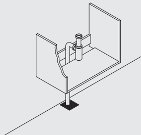
55 mm tila lattiaviemäröinnin putkille kaikissa allaskaapeissa.
