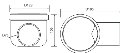
Vaakakaivo
