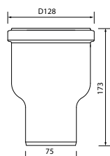
Pystykaivo
