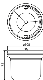
Erikoisvesilukko
